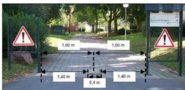
Dispositif filtrant sur une voie de largeur 3,2 m
